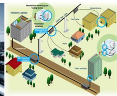
FTTH
